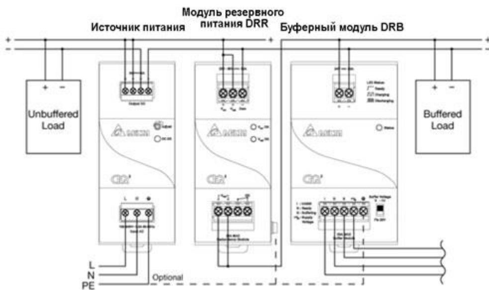
Схема с буферированием всей нагрузки и резервным питанием
