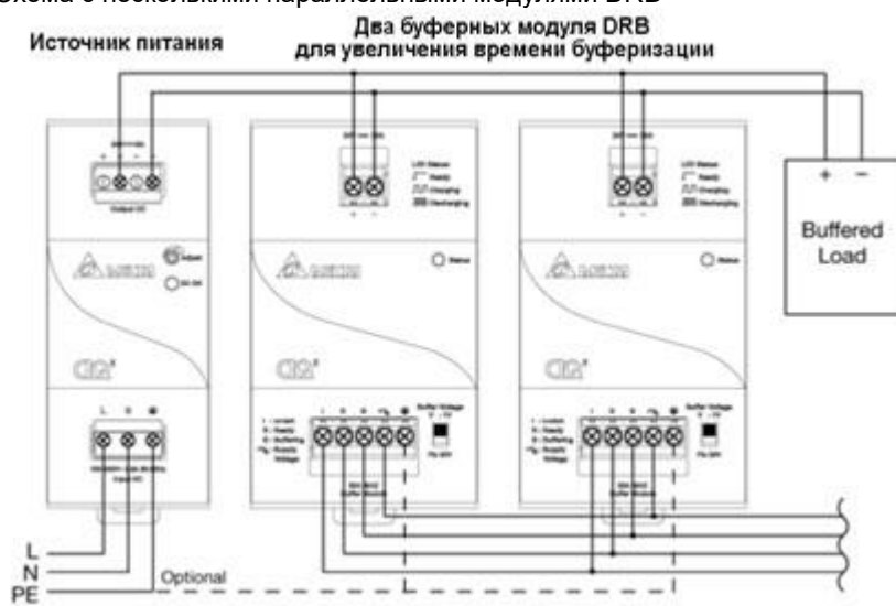
Схема с несколькими параллельными модулями DRB
