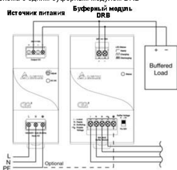
Схема с буферированием части нагрузки
