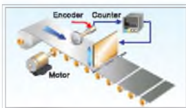
Система мерного реза
